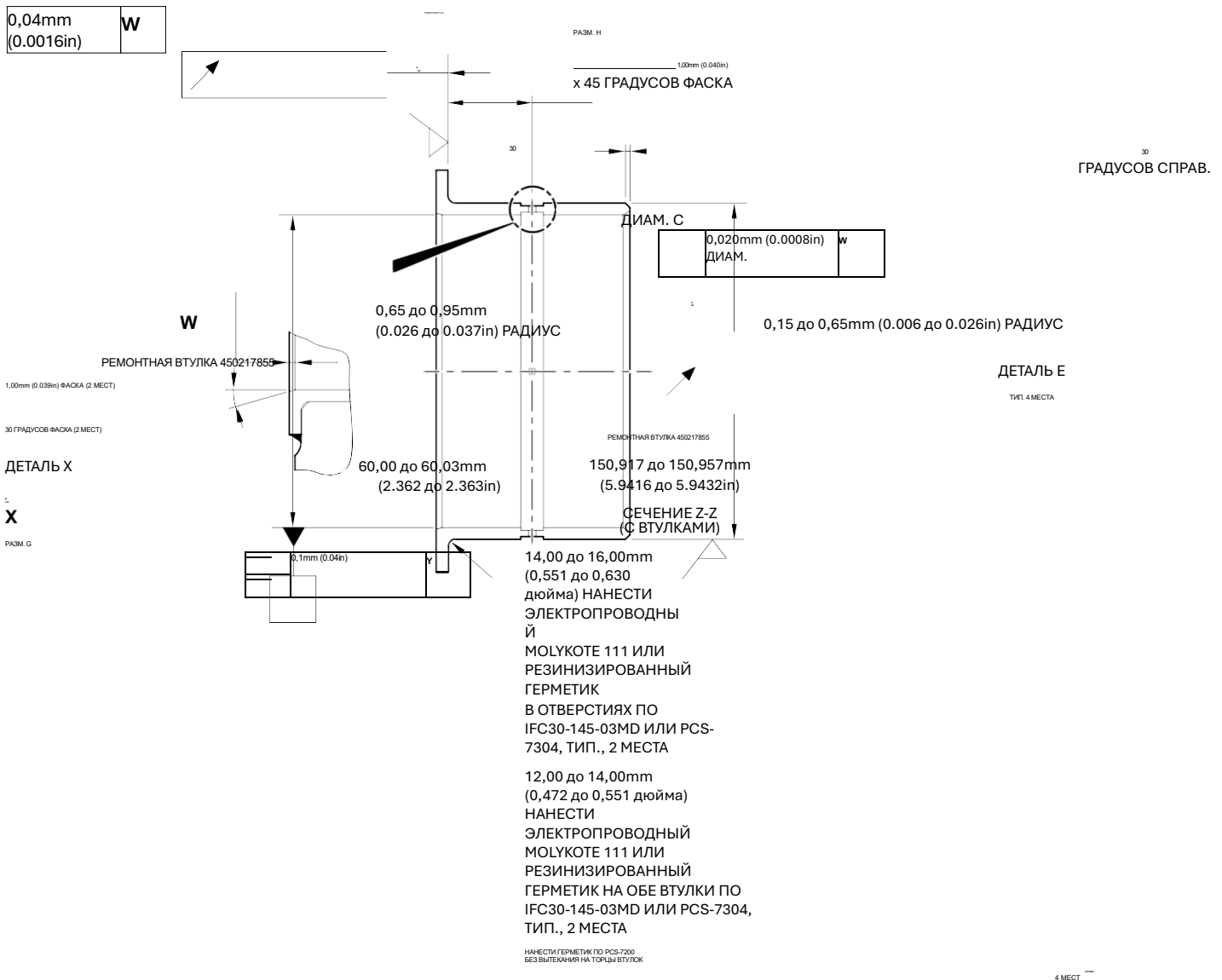
Ремонтные втулки — Механическая обработка и установка Рисунок 602
