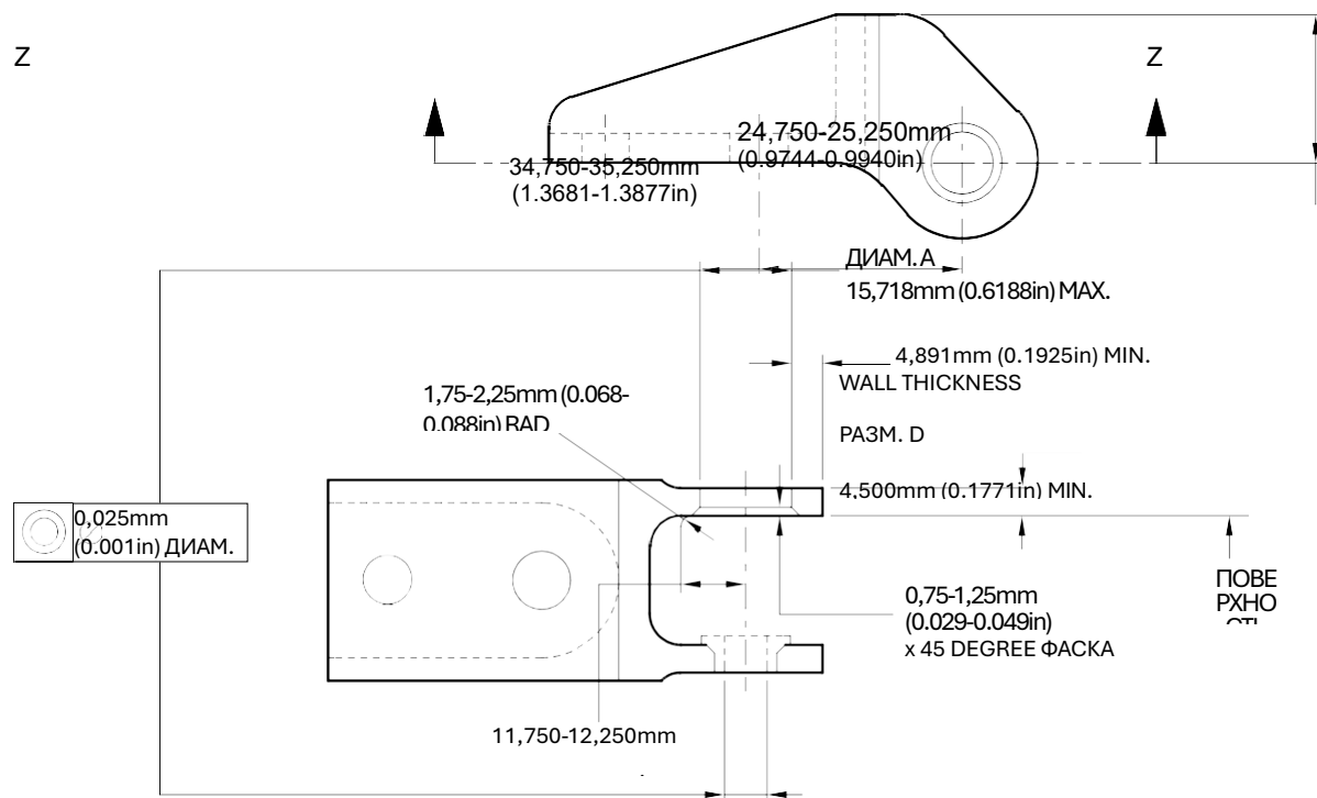
СЕЧЕНИЕ Z-Z WITHOUT ПОДШИПНИК
