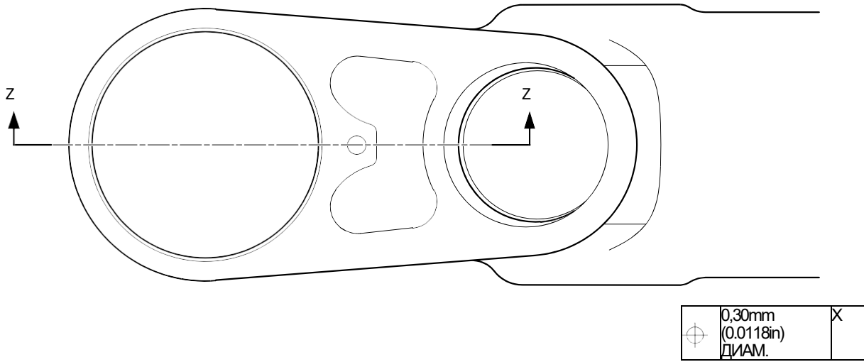
СЕЧЕНИЕ Z-Z (БЕЗ ПОДШИПНИКА)
