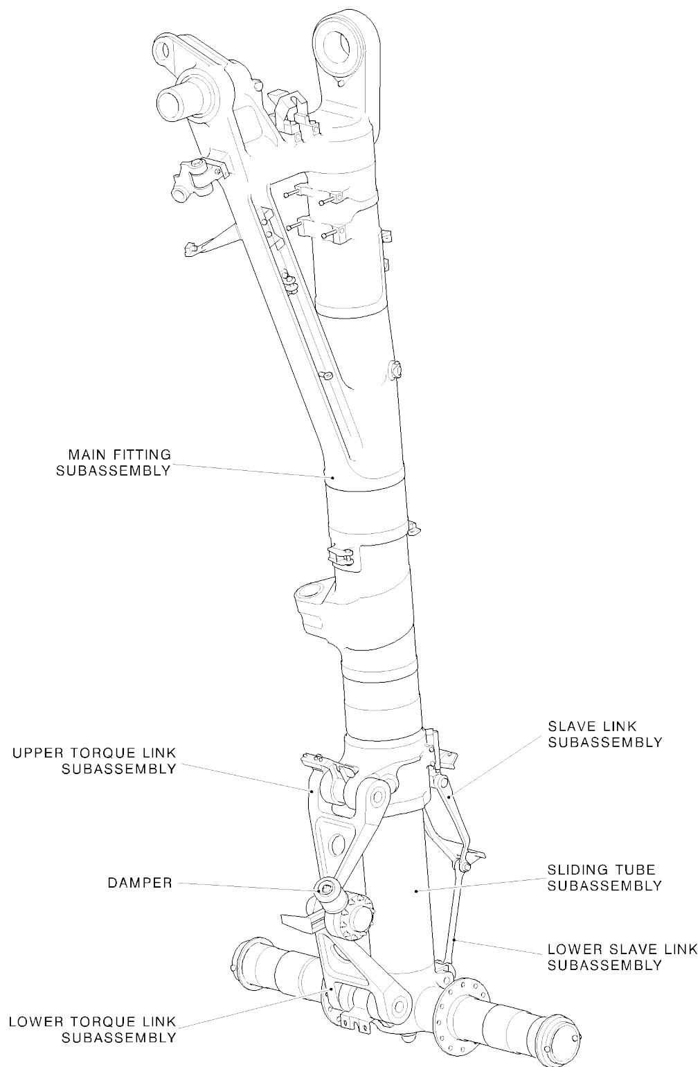
Стойка основного шасси рисунок 1
